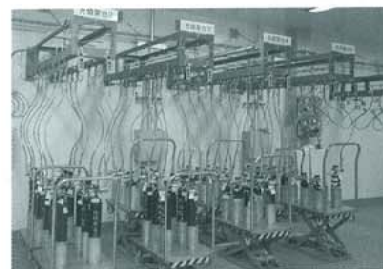
酸素ガス小瓶充てん台
